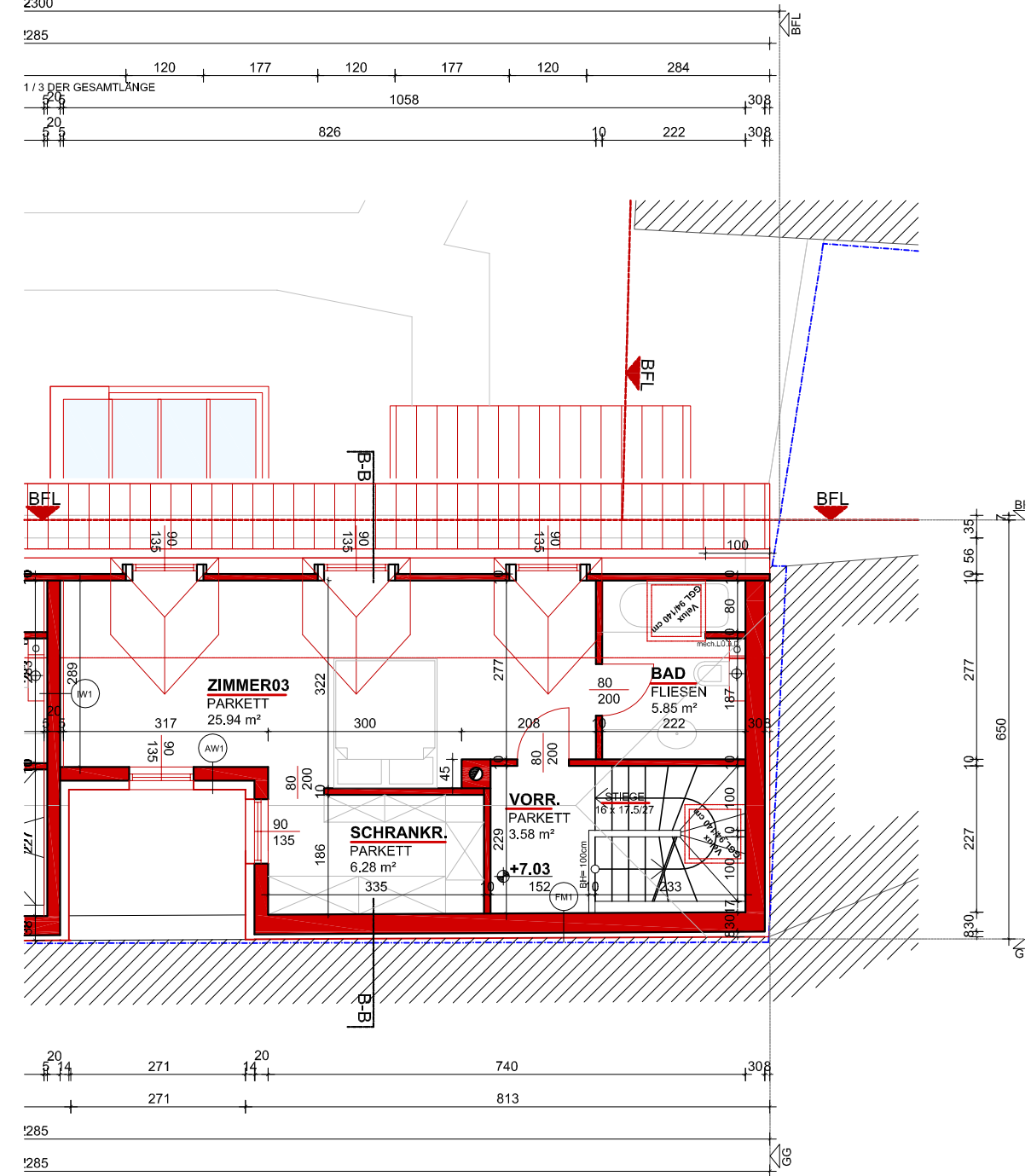
DACHGESCHOSS 1:100
