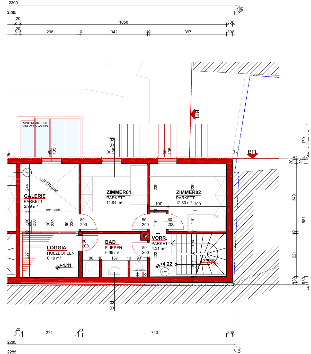
1. OBERGESCHOSS 1:100
