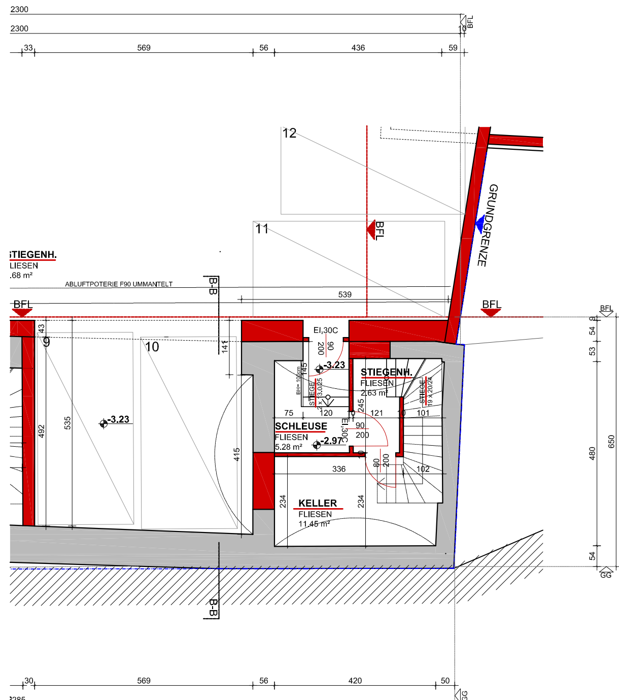
KELLERGESCHOSS 1:100
