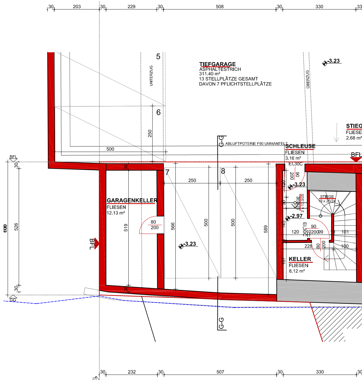
KELLERGESCHOSS 1:100
