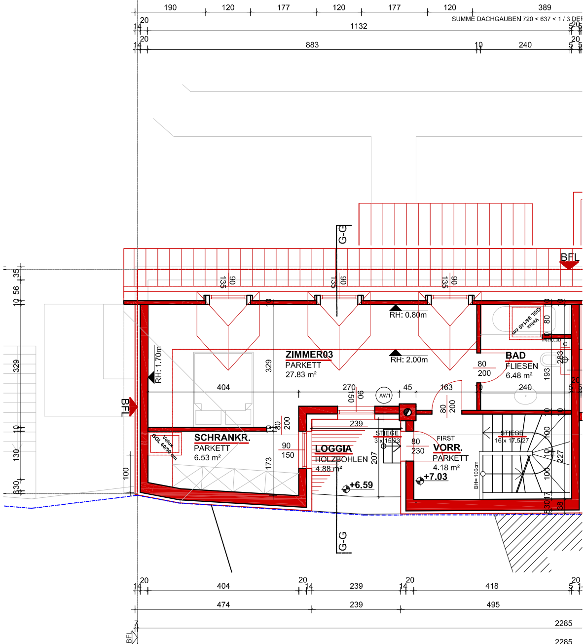
DACHGESCHOSS 1:100
