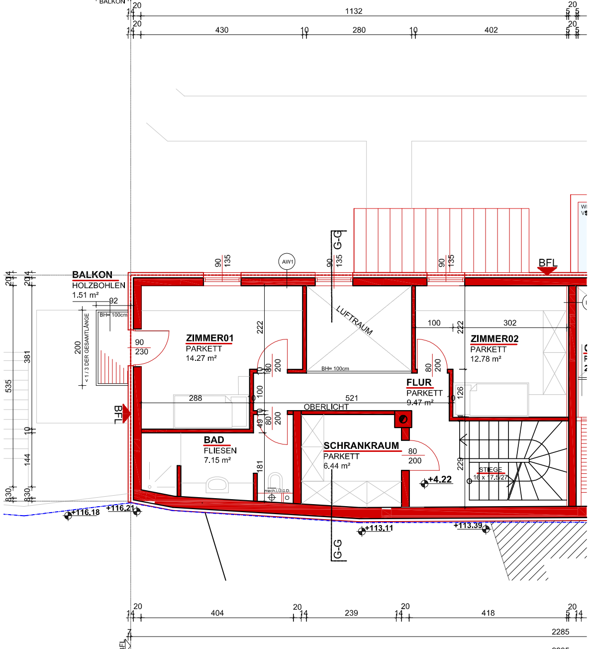
1. OBERGESCHOSS 1:100
