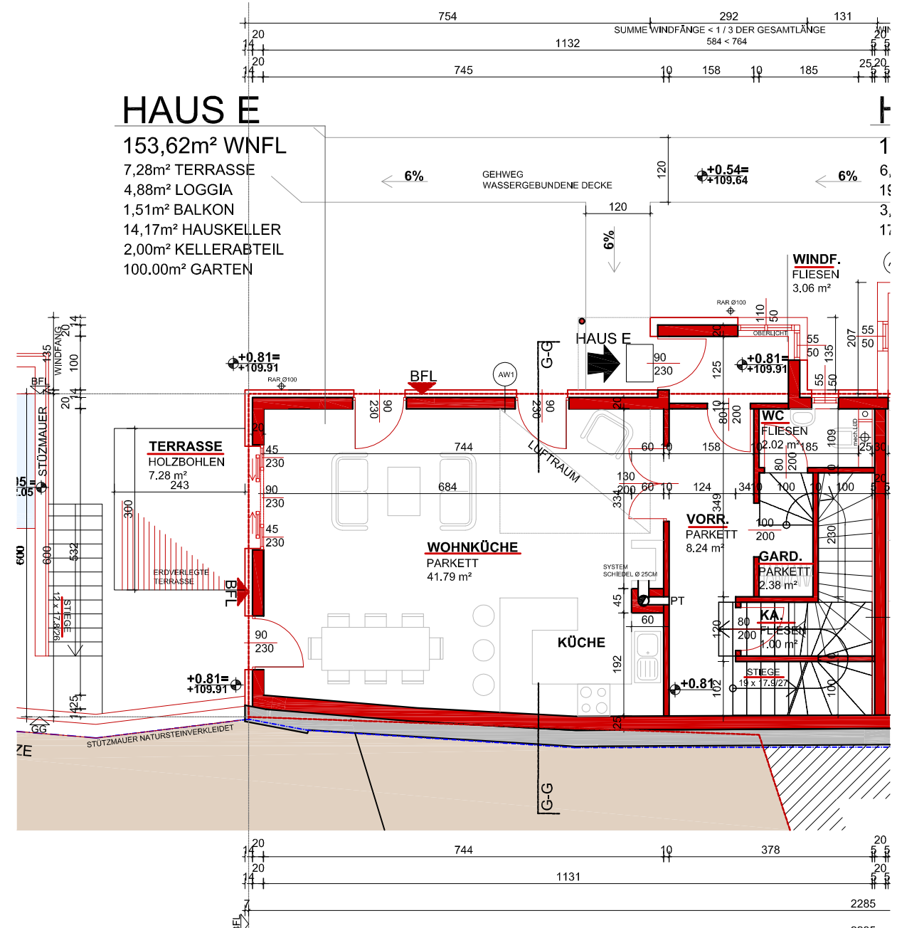
ERDGESCHOSS 1:100
