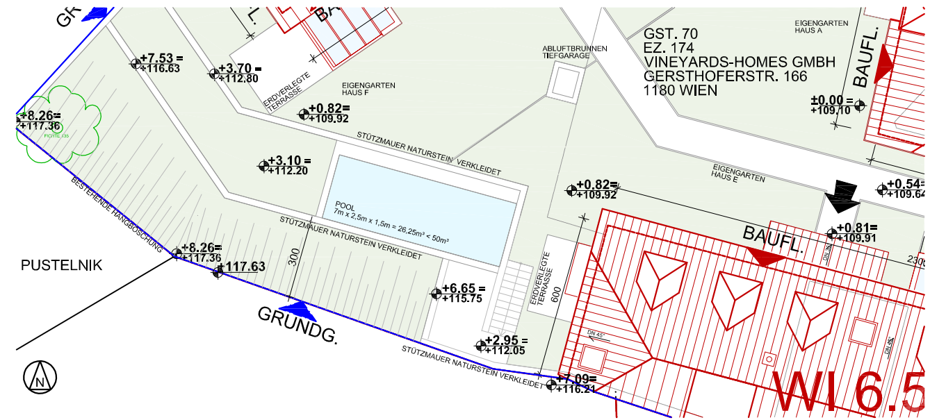
LAGEPLAN 1:500
