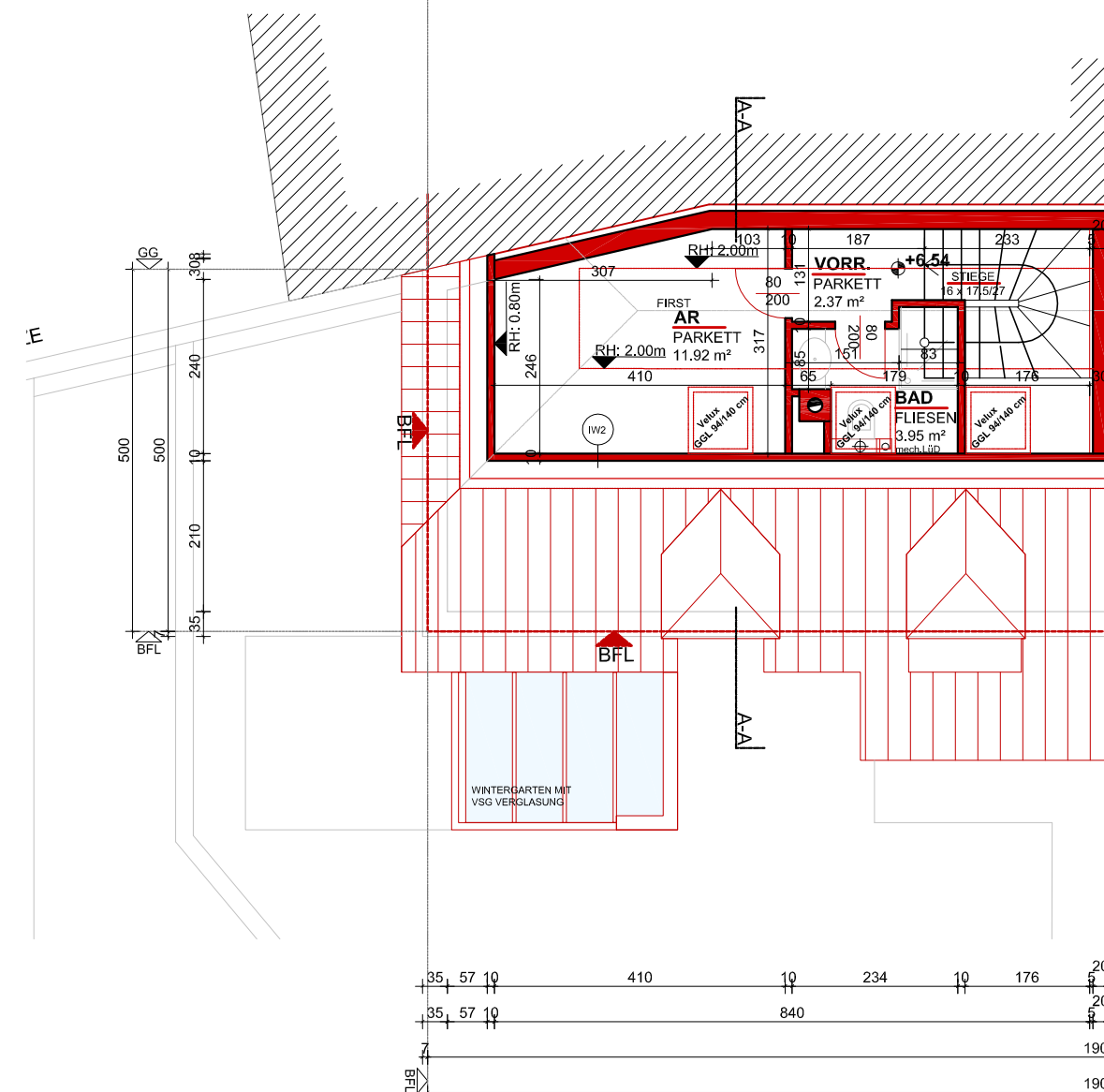
DACHGESCHOSS 1:100
