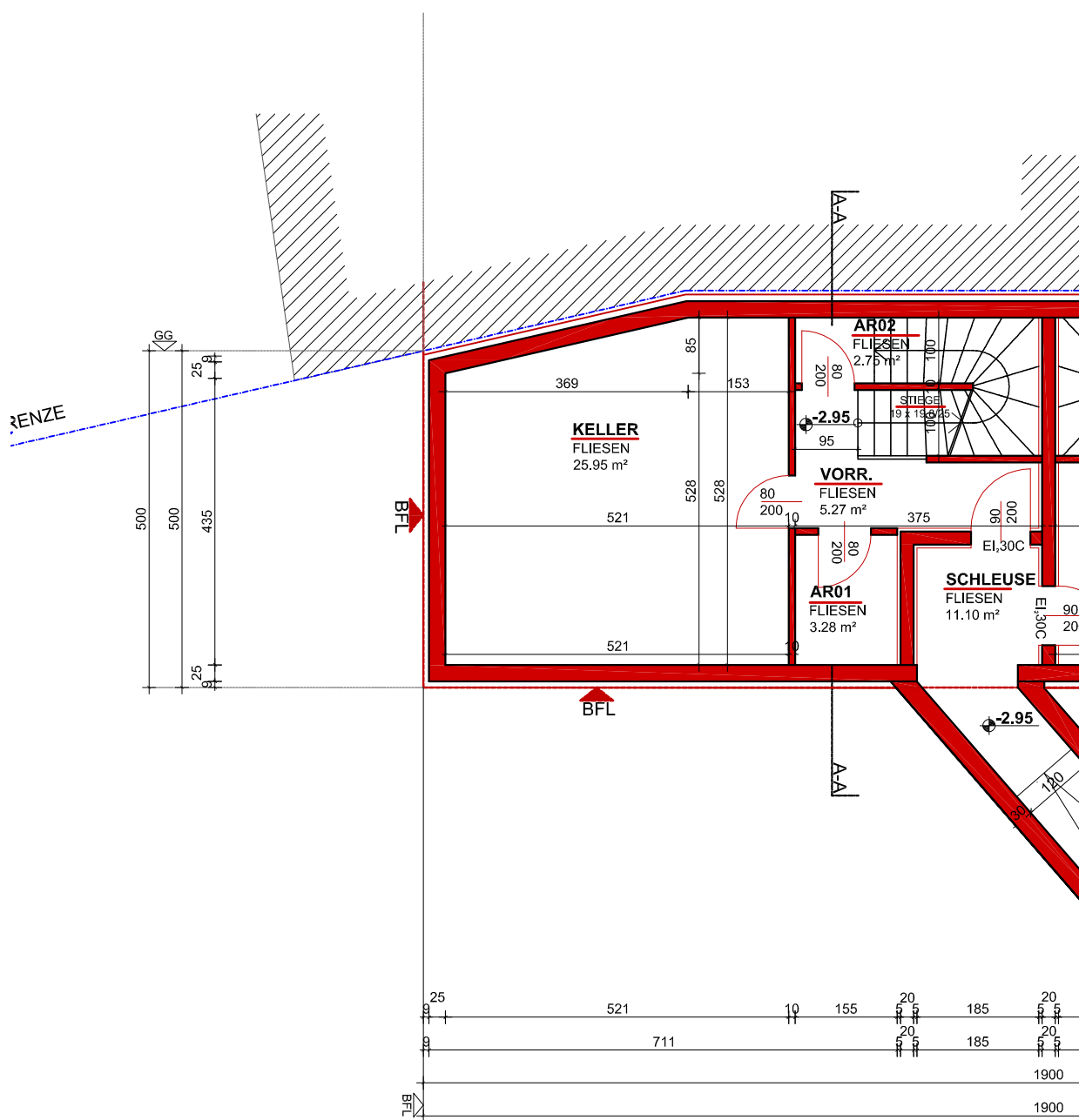
KELLERGESCHOSS 1:100
