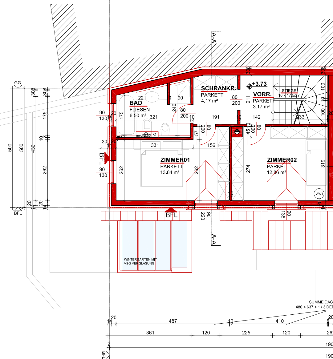
1. OBERGESCHOSS 1:100
