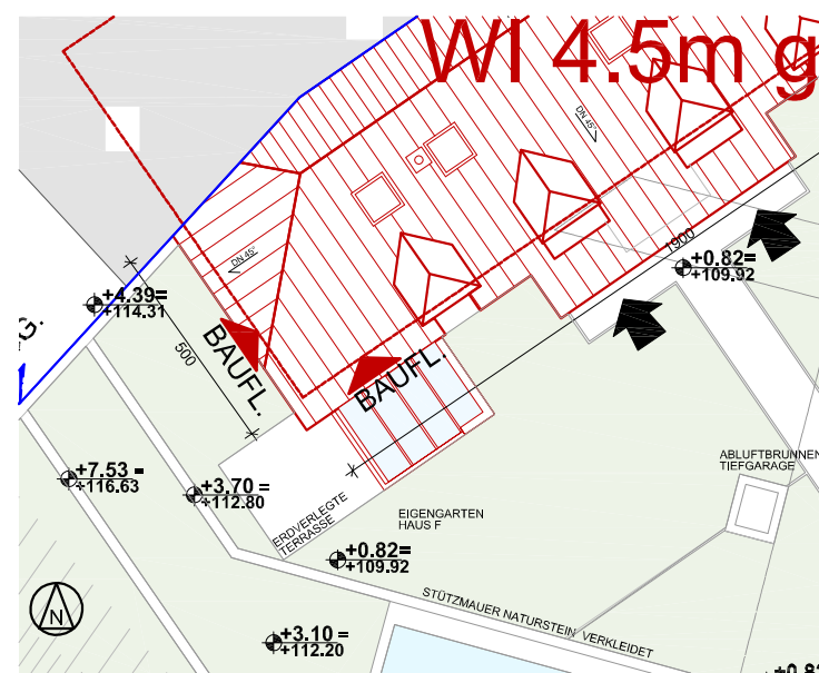
LAGEPLAN 1:500
