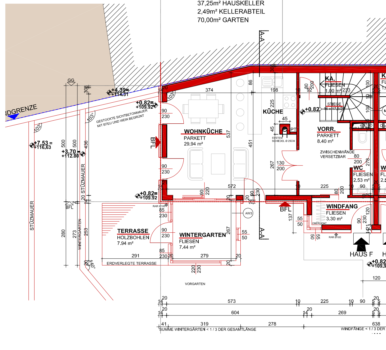
ERDGESCHOSS 1:100
