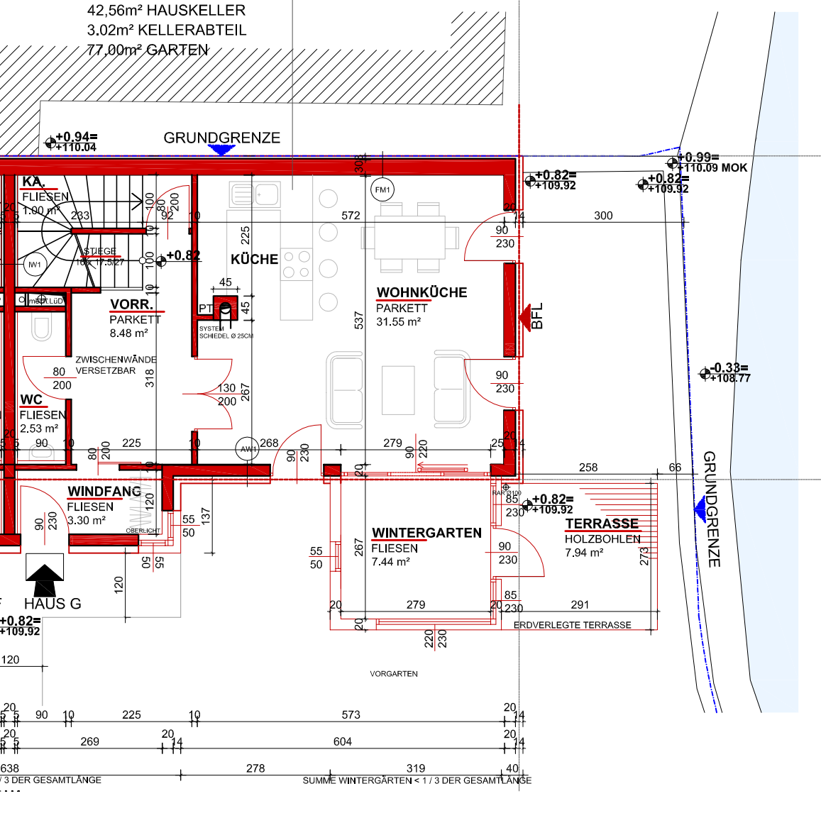
ERDGESCHOSS 1:100
