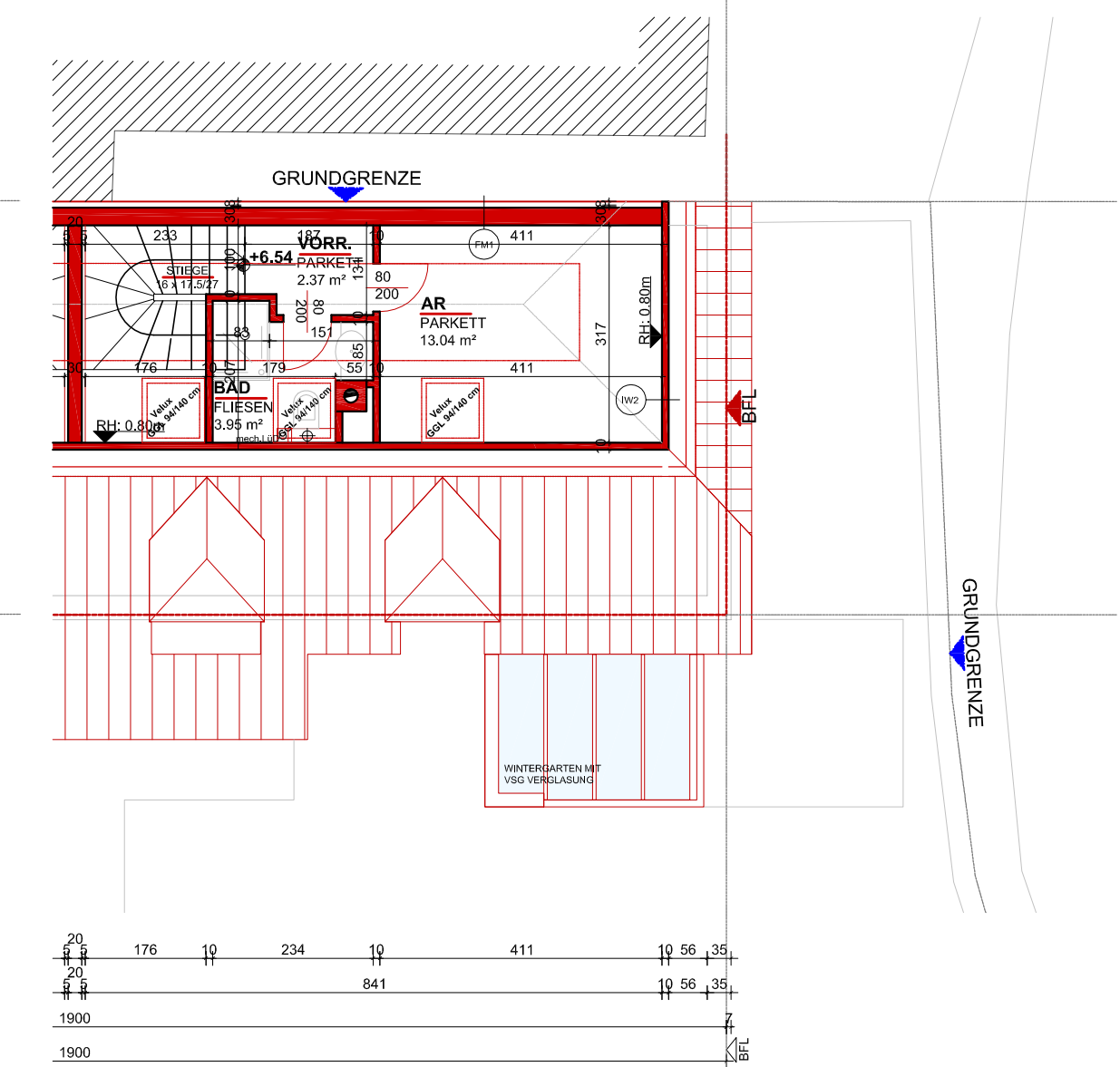
DACHGESCHOSS 1:100
