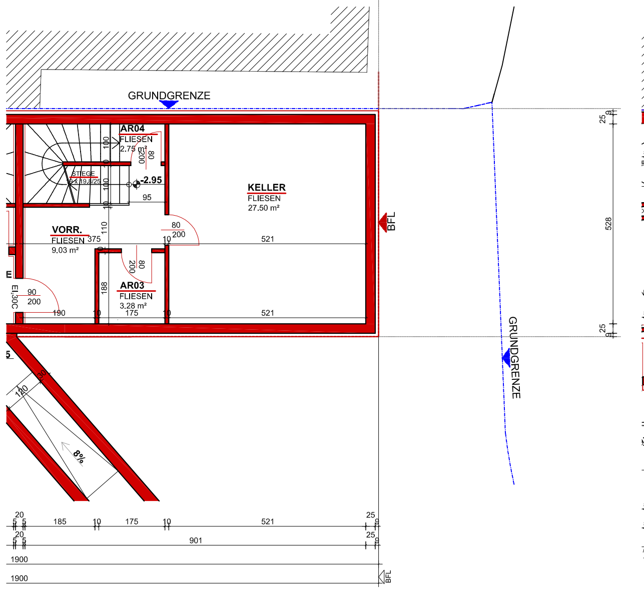
KELLERGESCHOSS 1:100
