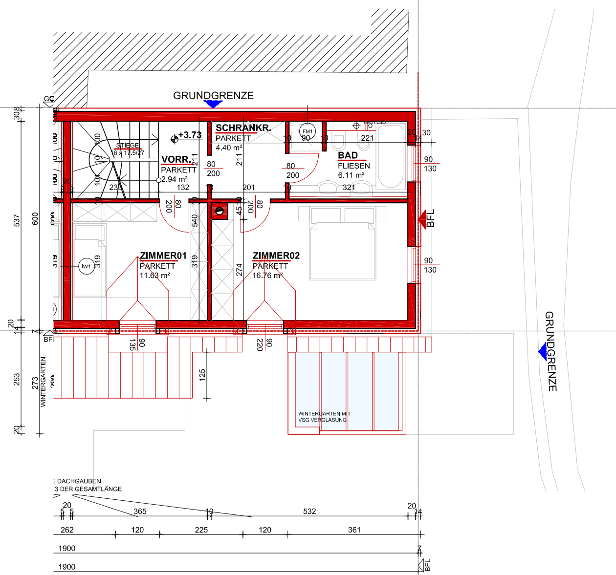
1. OBERGESCHOSS 1:100
